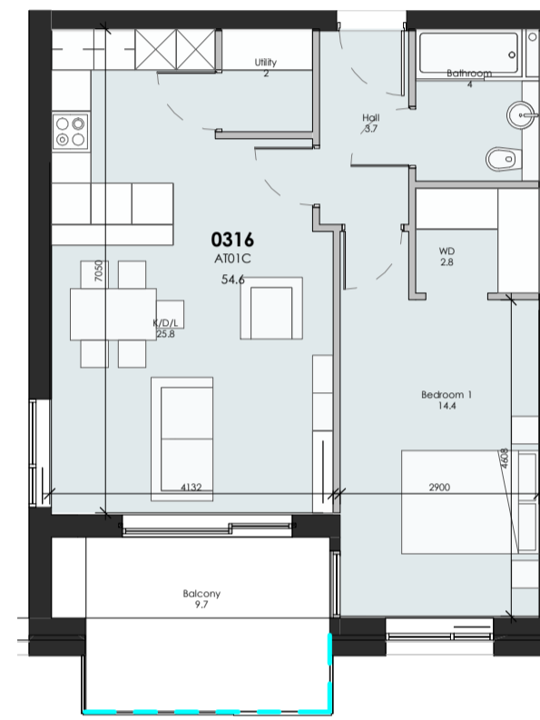
③ AT01C 1:100
