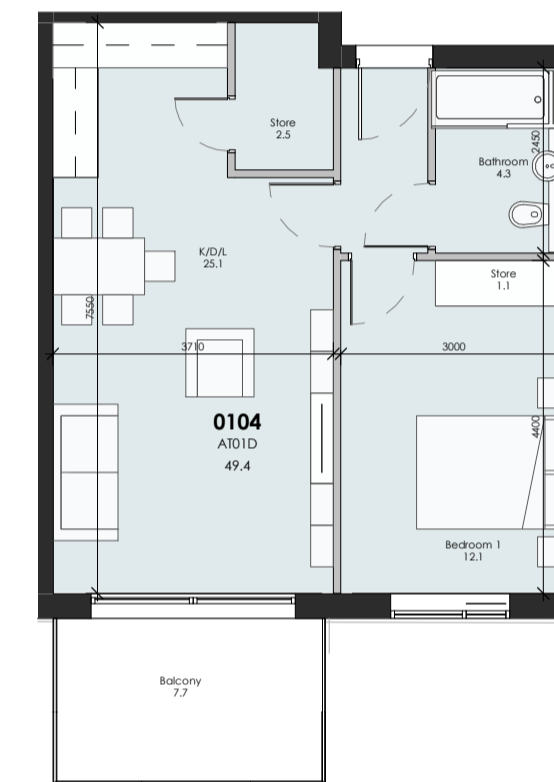
④ AT01D 1:100
