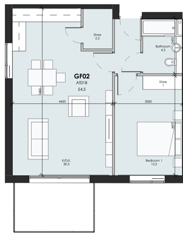
① AT01B 1:100
