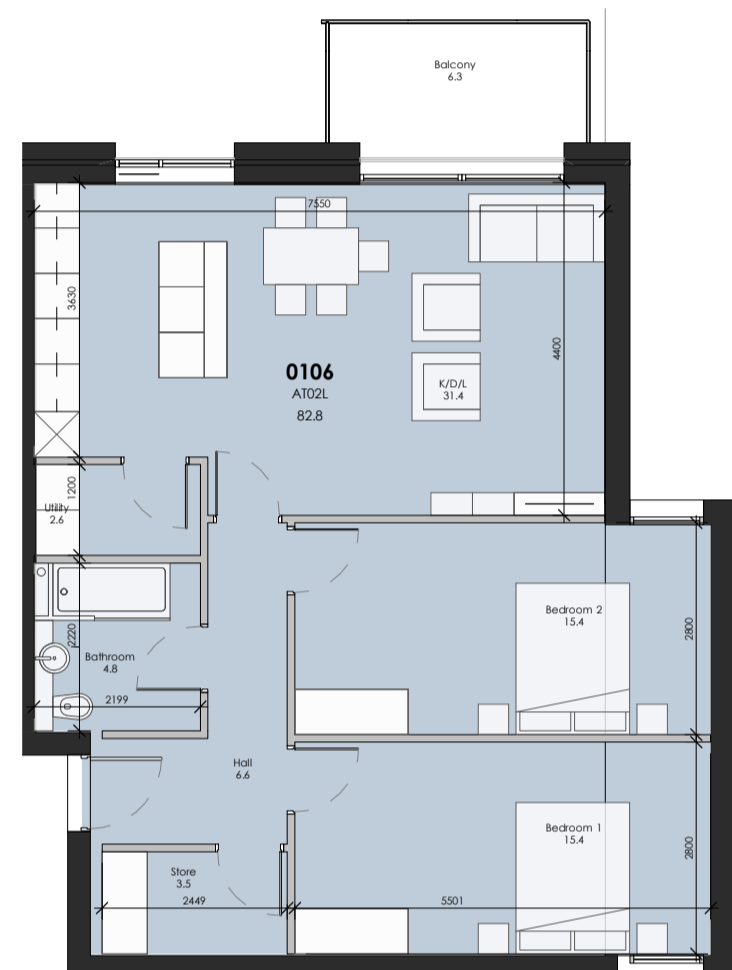
① AT02L 1:100
